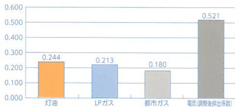
エネルギー別二酸化炭素排出係数 (kg-CO 2 /kWh)
